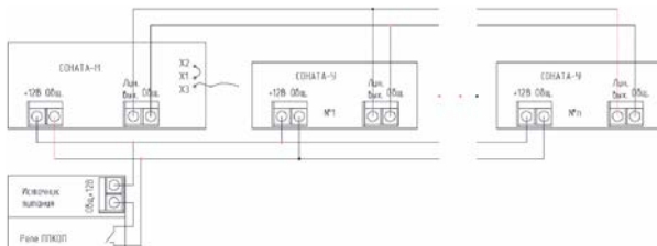
Рисунок 3. Подключение оповещателей СОНАТА-У к оповещателю СОНАТА-М.
