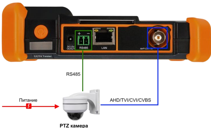
Рис.7 Подключение управляемой PTZ видеокамеры к тестеру
