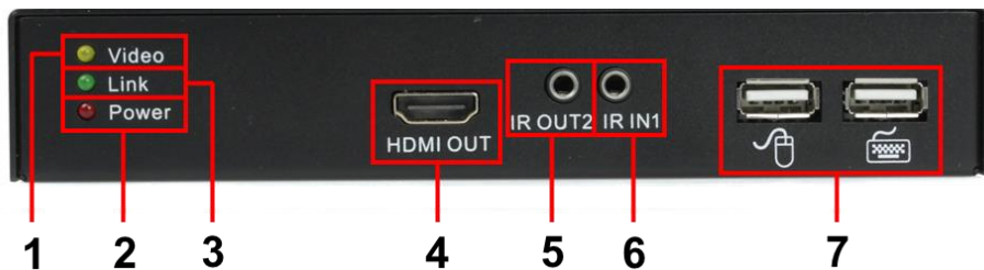
Рис. 4 Приемник RA-NiKM, разъемы и индикаторы на передней панели
