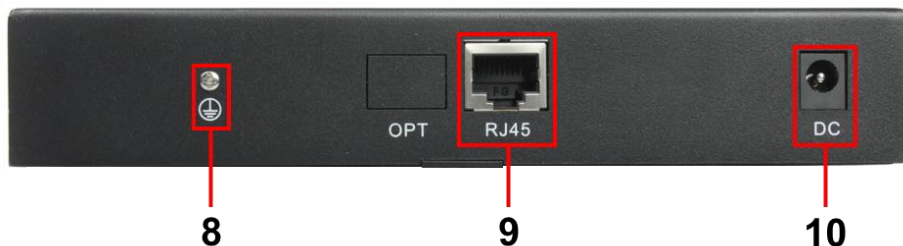
Рис. 5 Приемник RA-NiKM, разъемы и индикаторы на задней панели
