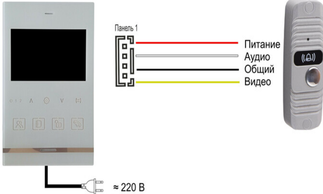
Рис. Минимальная система видеодомофона без управления замком
