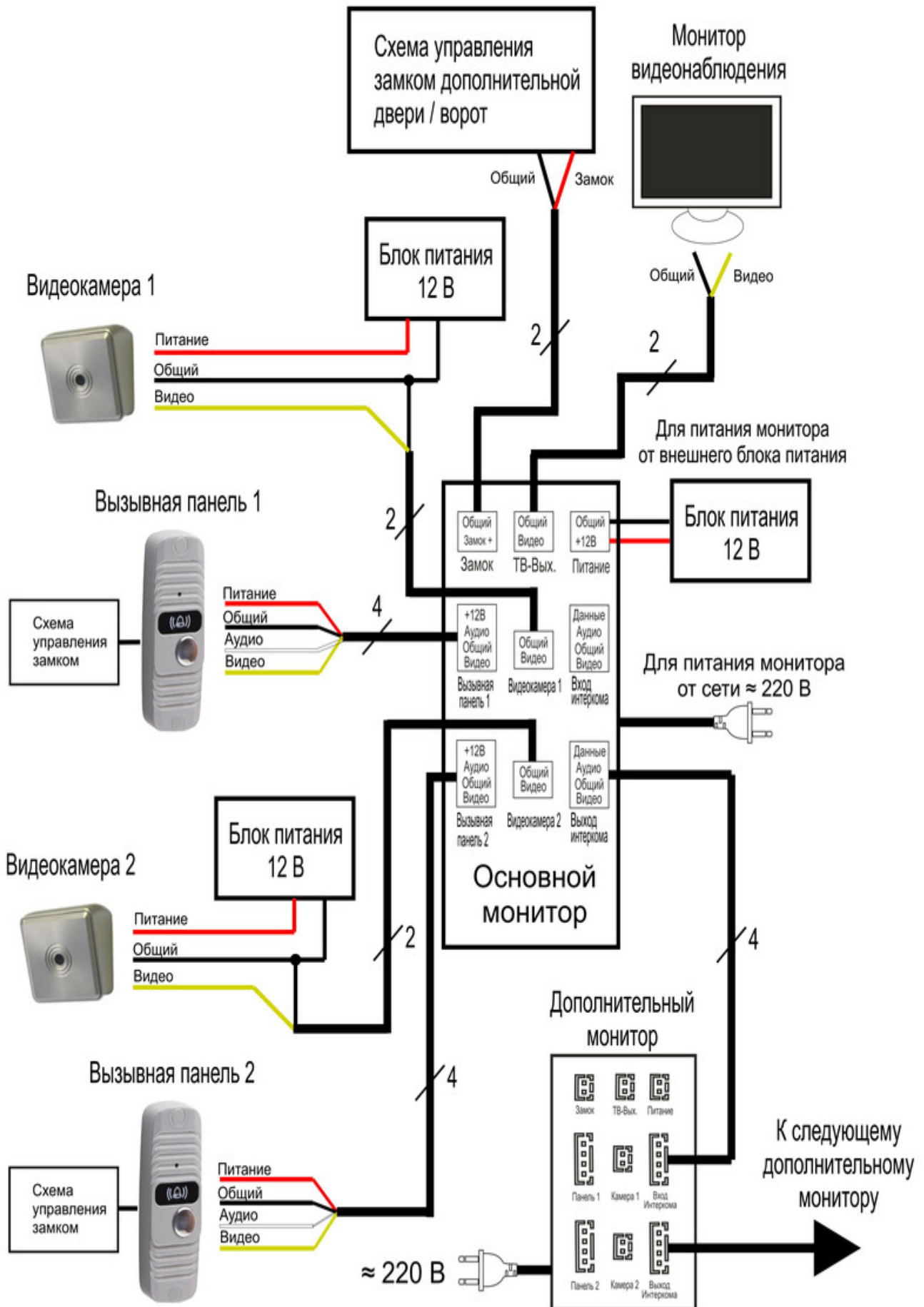
Рис. Общая схема подключения монитора
