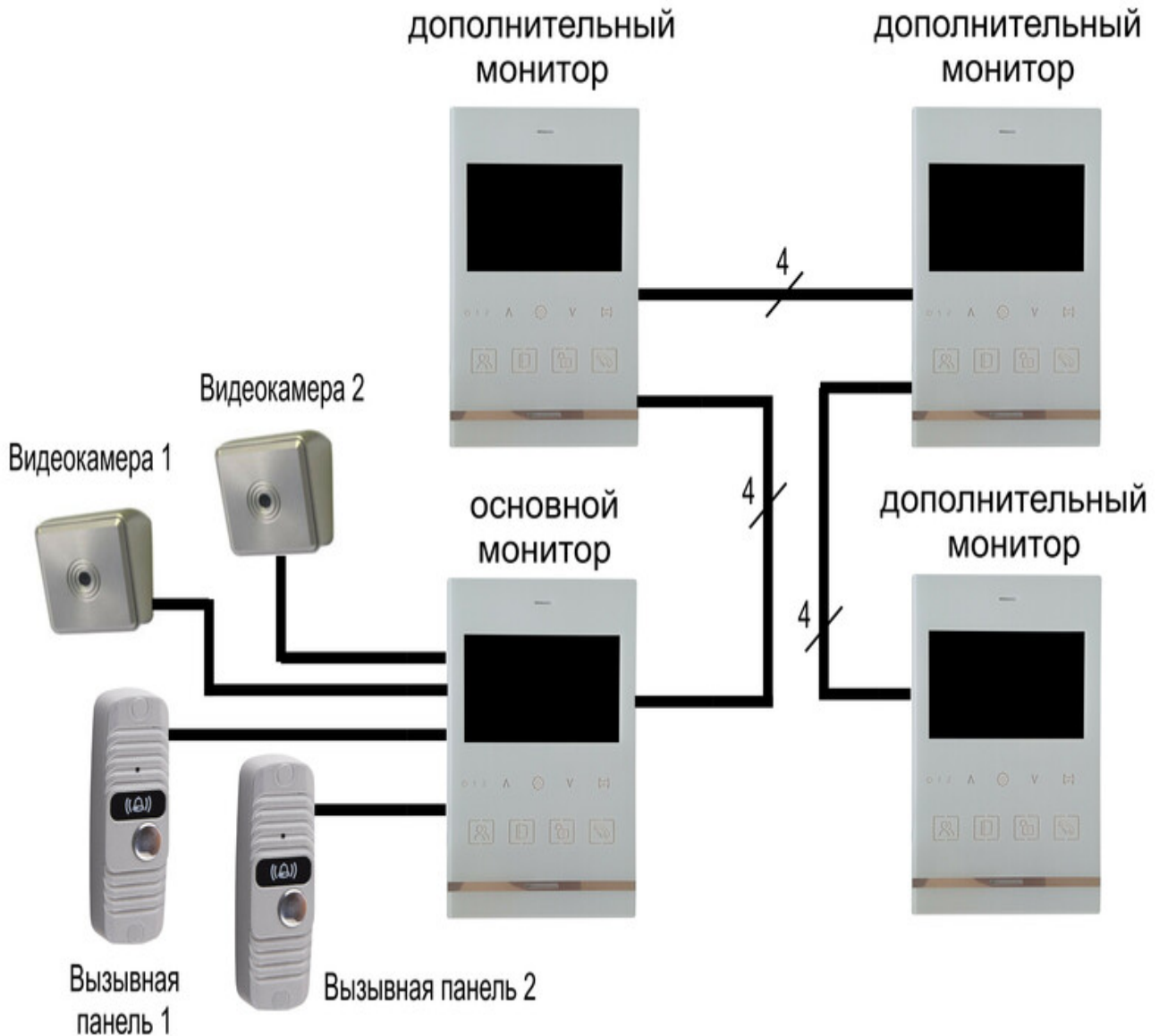
Рис. Схема подключения мониторов в режиме интеркома
