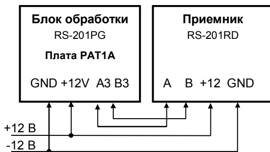
Рис. 2. Подключение приемника RS-201RD к блоку обработки
