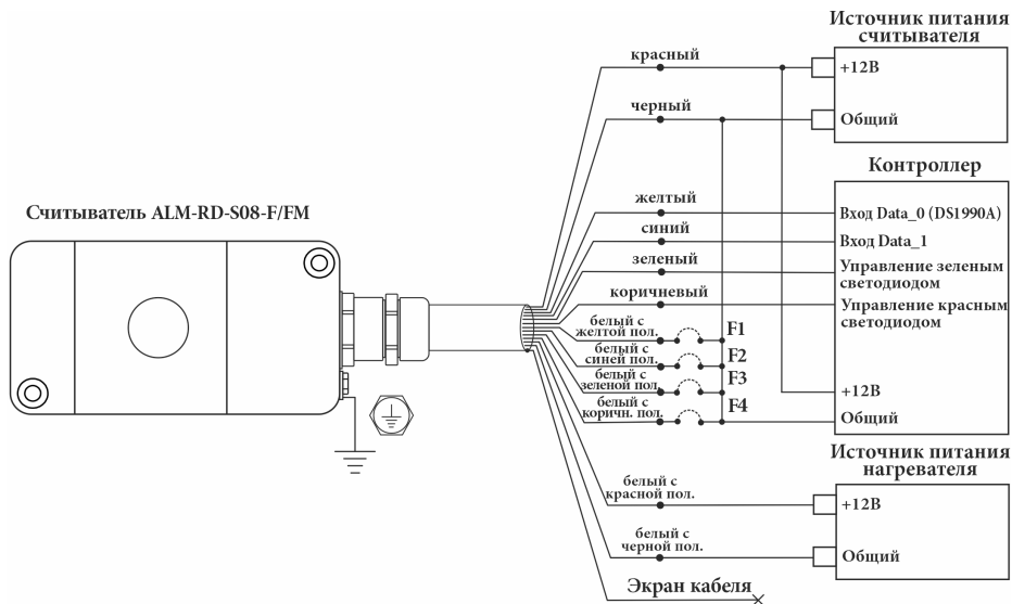
Рисунок 3 – Схема подключения счетчика ALM-RD-S08-F/FM к контроллеру СКУД с разделным питанием счетчика и нагревателя
