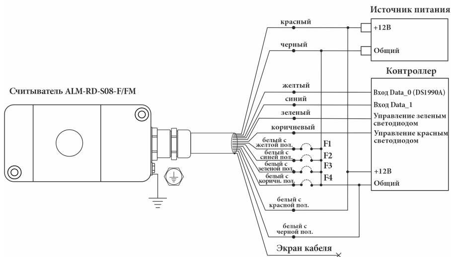
Рисунок 4 – Схема подключения счетчика ALM-RD-S08-F/FM к контроллеру СКУД с питанием счетчика и нагревателя от одного источника питания.
