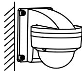
DS-1258ZJ Кронштейн для установки на стену
